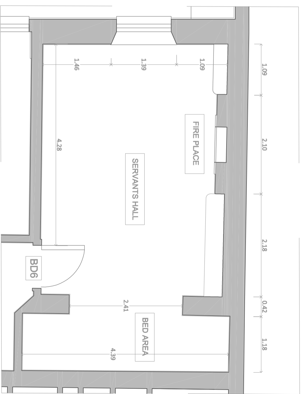
Servants Hall. Floorplan. 1:50 (meters)
